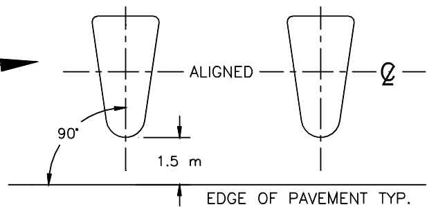
DETAIL-2 EDGE MOUNT
